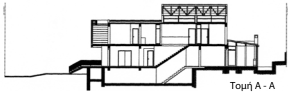
Τομή Α - Α
